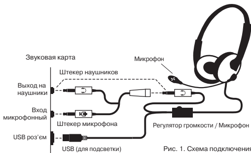
Рис. 1. Схема подключения
