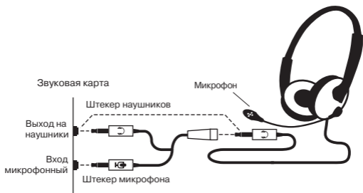
Рис. 1. Схема подключения
