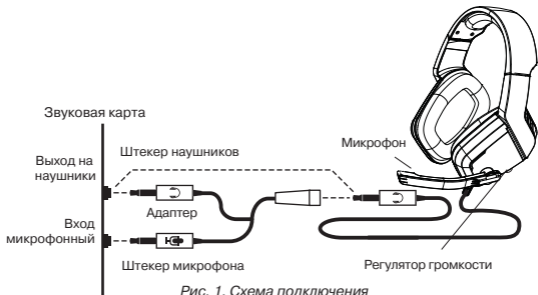
Рис. 1. Схема подключения
