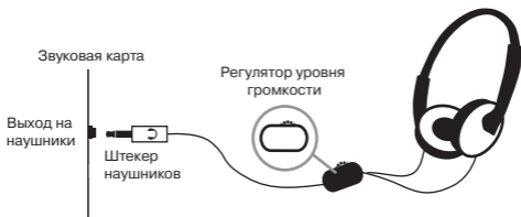
Рис. 1. Схема подключения
