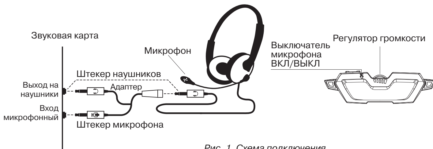
Рис. 1. Схема подключения
