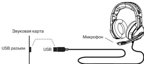
Рис. 1. Схема подключения
