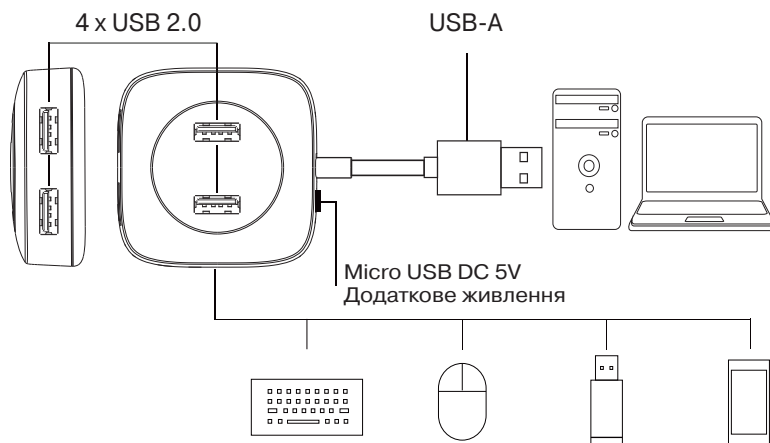
Схема підключення
