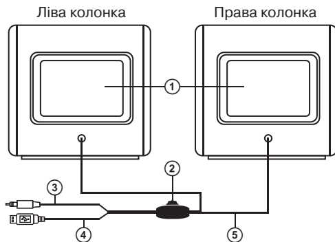
Мал. 1. Задні панелі колонок
