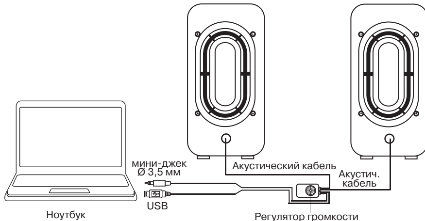
Рис. 3. Схема подключения
