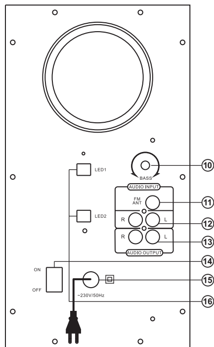
Рис. 2. Задняя панель сабвуфера
