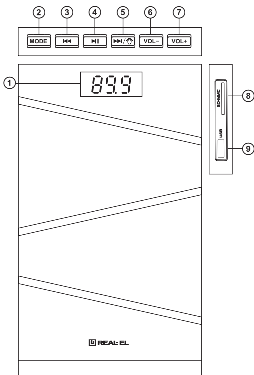
Рис. 1. Панель управления сабвуфера
