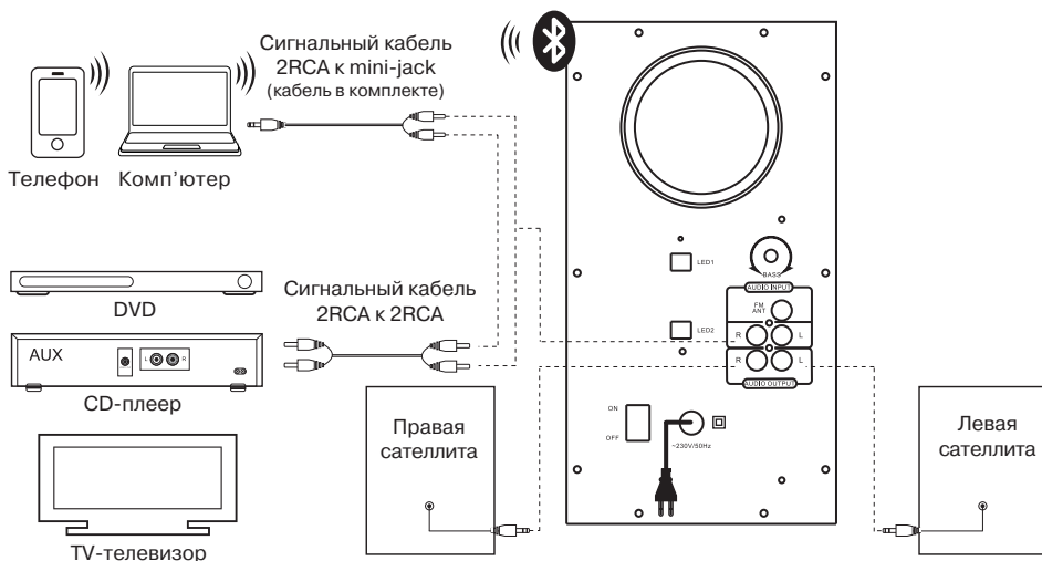
Рис. 5. Схема подключения
