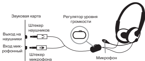
Рис. 1. Схема подключения
